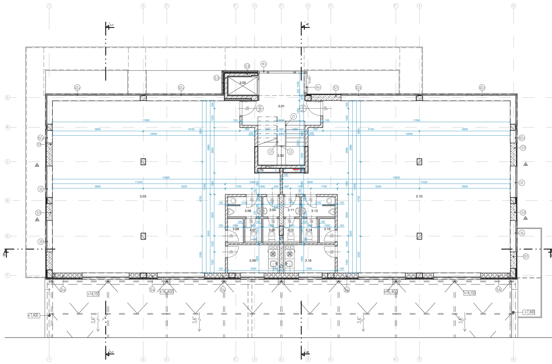
PÔDORYS 3. NADZEMNÉHO PODLAŽIA M 1:100
