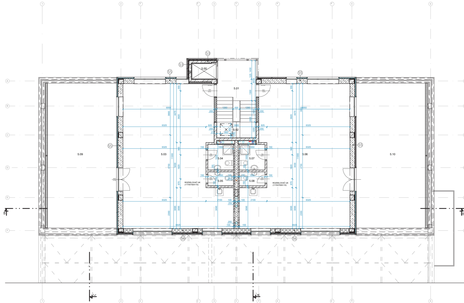
PÔDORYS 5. NADZEMNÉHO PODLAŽIA M 1:100
